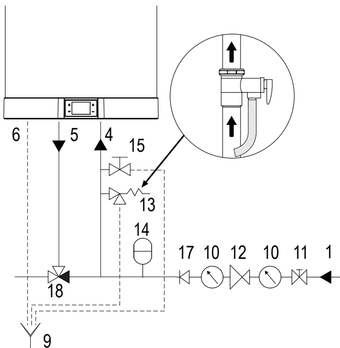
fig. 57 - Exemple installation hydraulique
