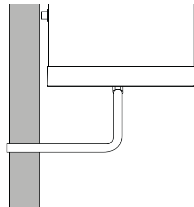
fig. 58 - Exemples de raccordement de l'évacuation des condensats sans siphon
