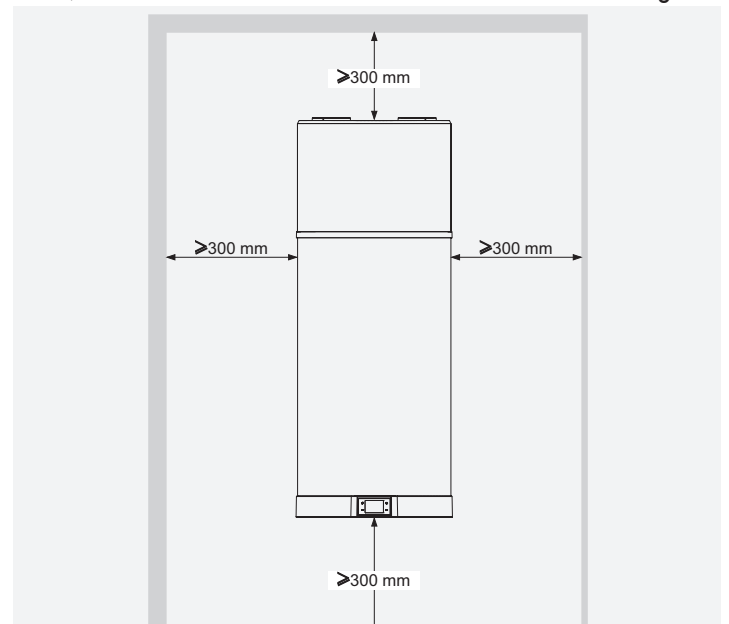
fig. 49 - Espaços mínimos
