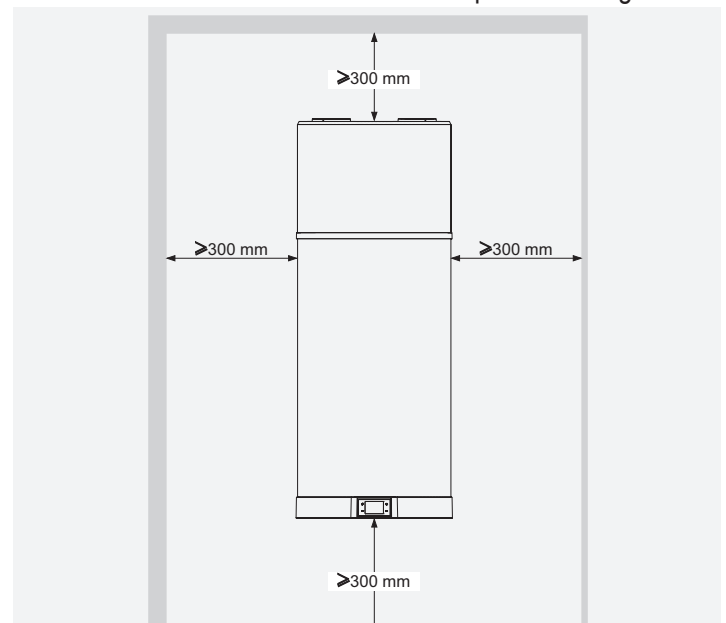
fig. 49 - Espaces minimum
