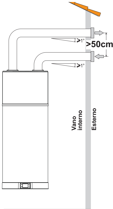
fig. 54 - Exemplo de ligação de descarga de ar
