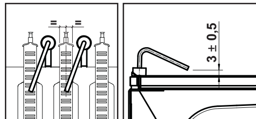
fig. 13 - Colocação dos eléctrodos
