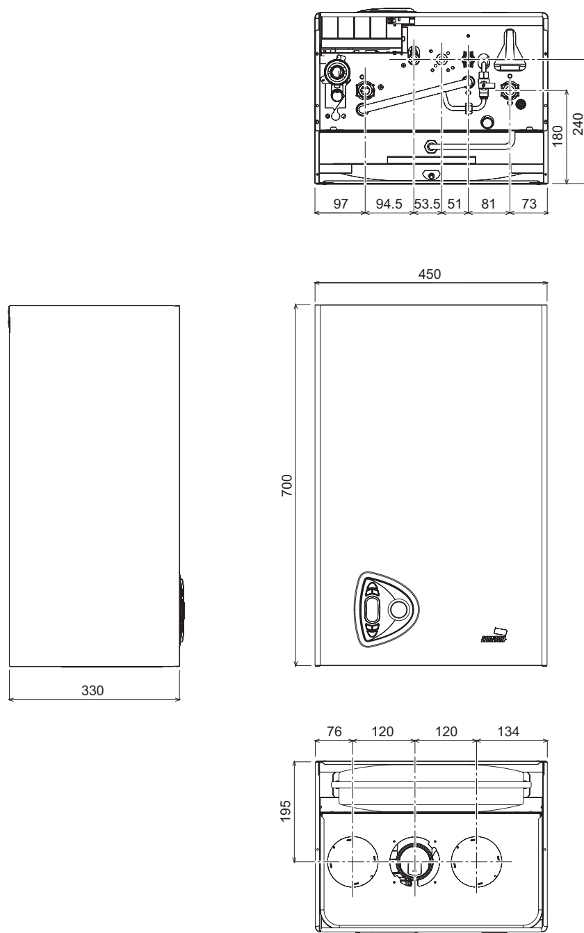
fig. 30 - Dimensiones y conexiones
