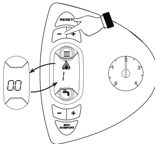
fig. 13 - Modalidad TEST (potencia de la calefacción = 100%)
