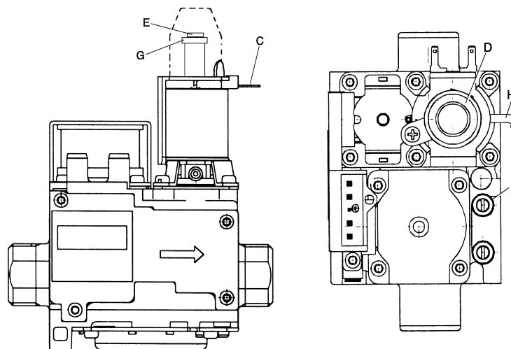
fig. 14 - Válvula del gas
