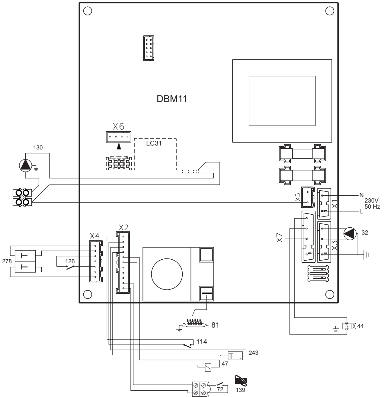
fig. 19 - Esquema eléctrico
