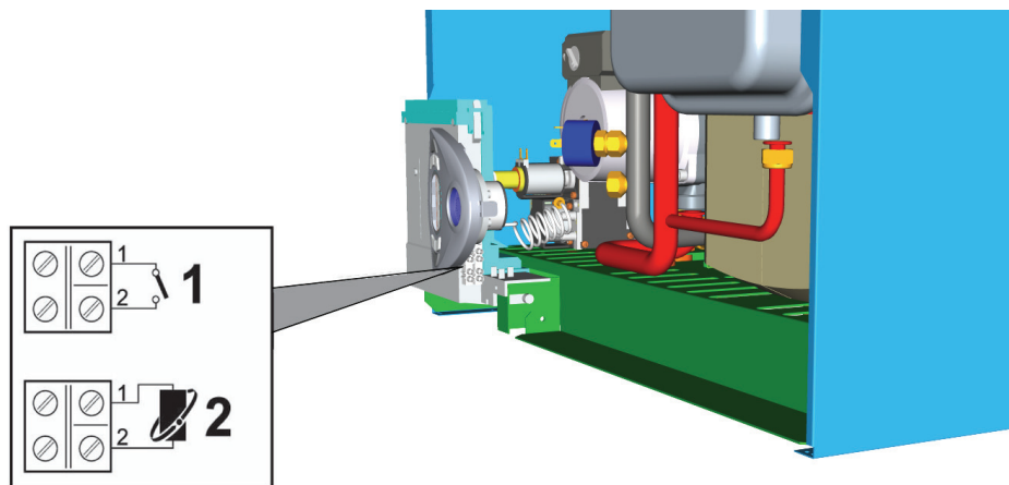
fig. 12 - Acceso a la regleta de conexiones
