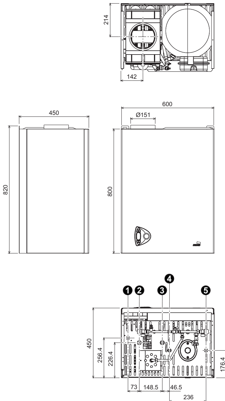
fig. 16 - Dimensiones y conexiones
