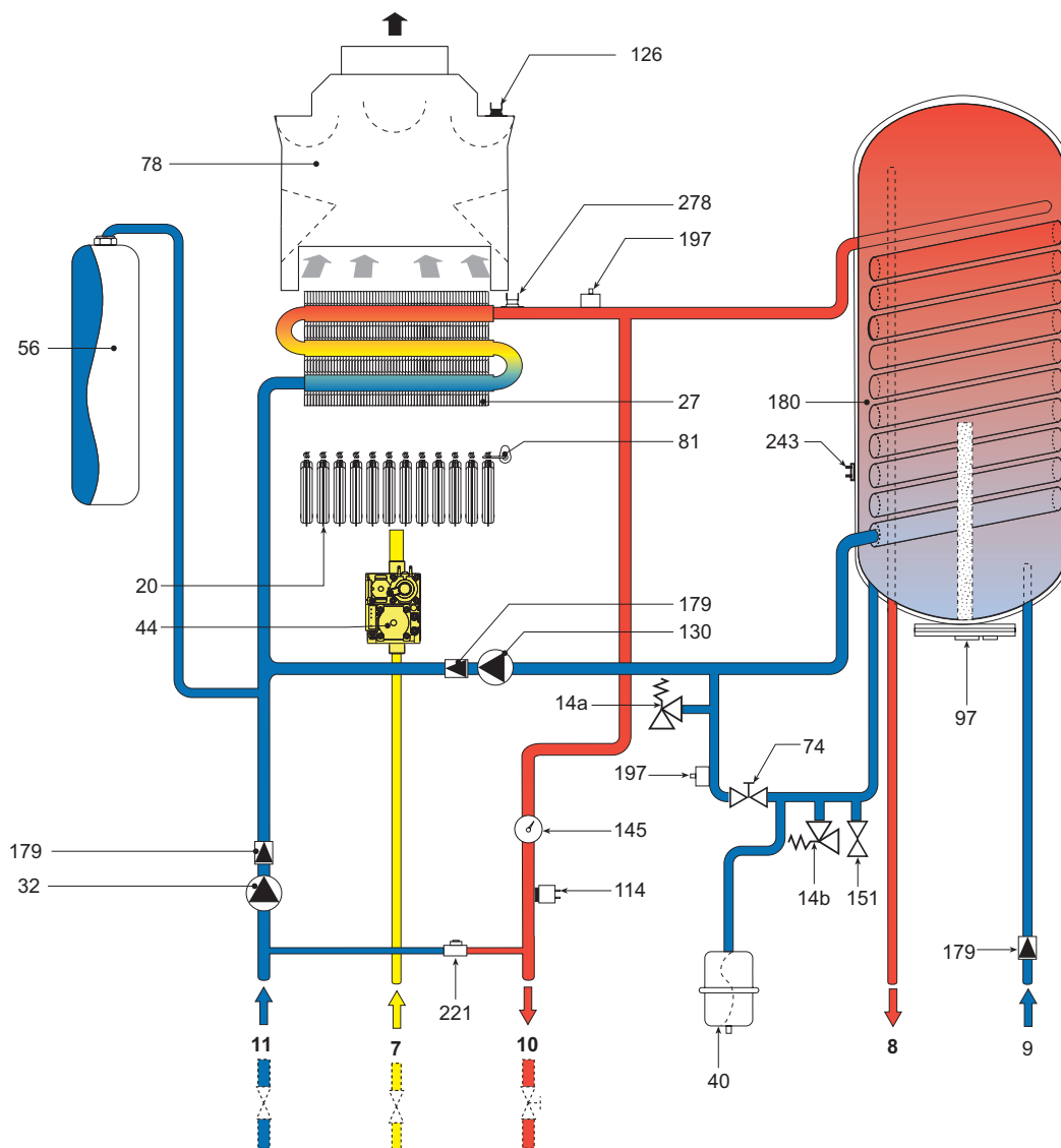
fig. 18 - Circuito hidráulico
