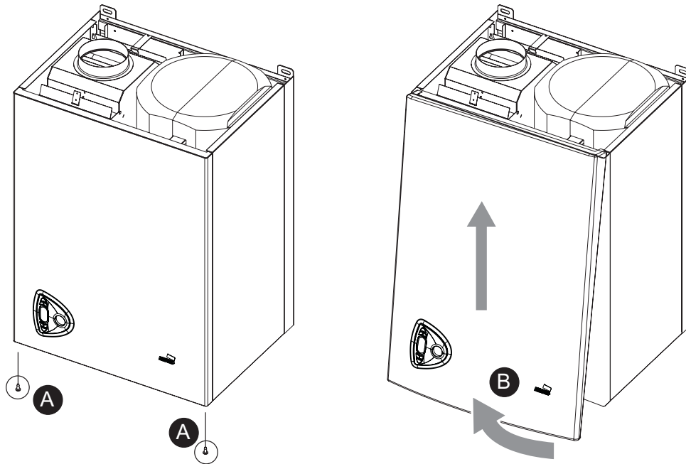
fig. 15 - Apertura de la carcasa
