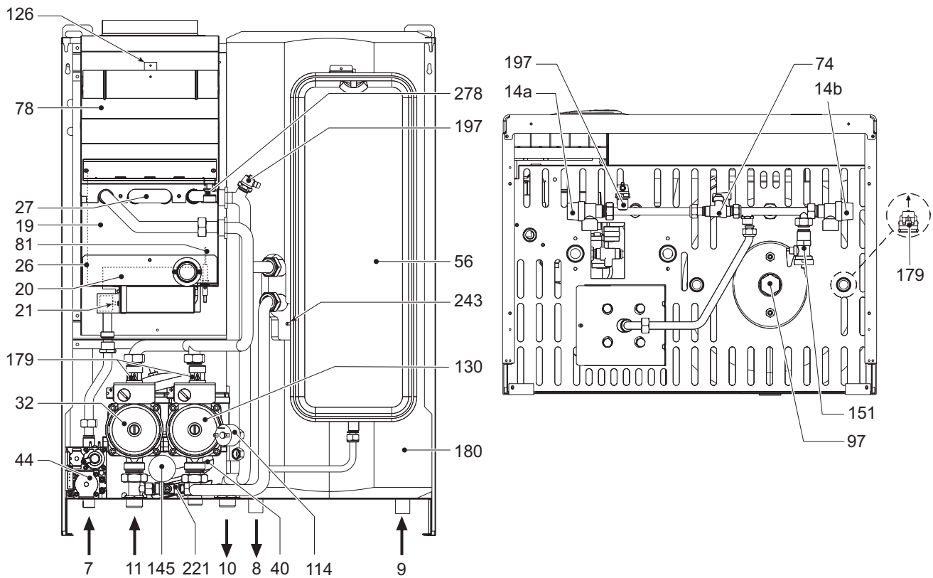
fig. 17 - Vista general
