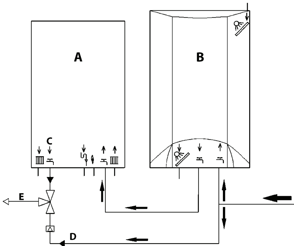
fig. 18 - Esquema de instalación solar
