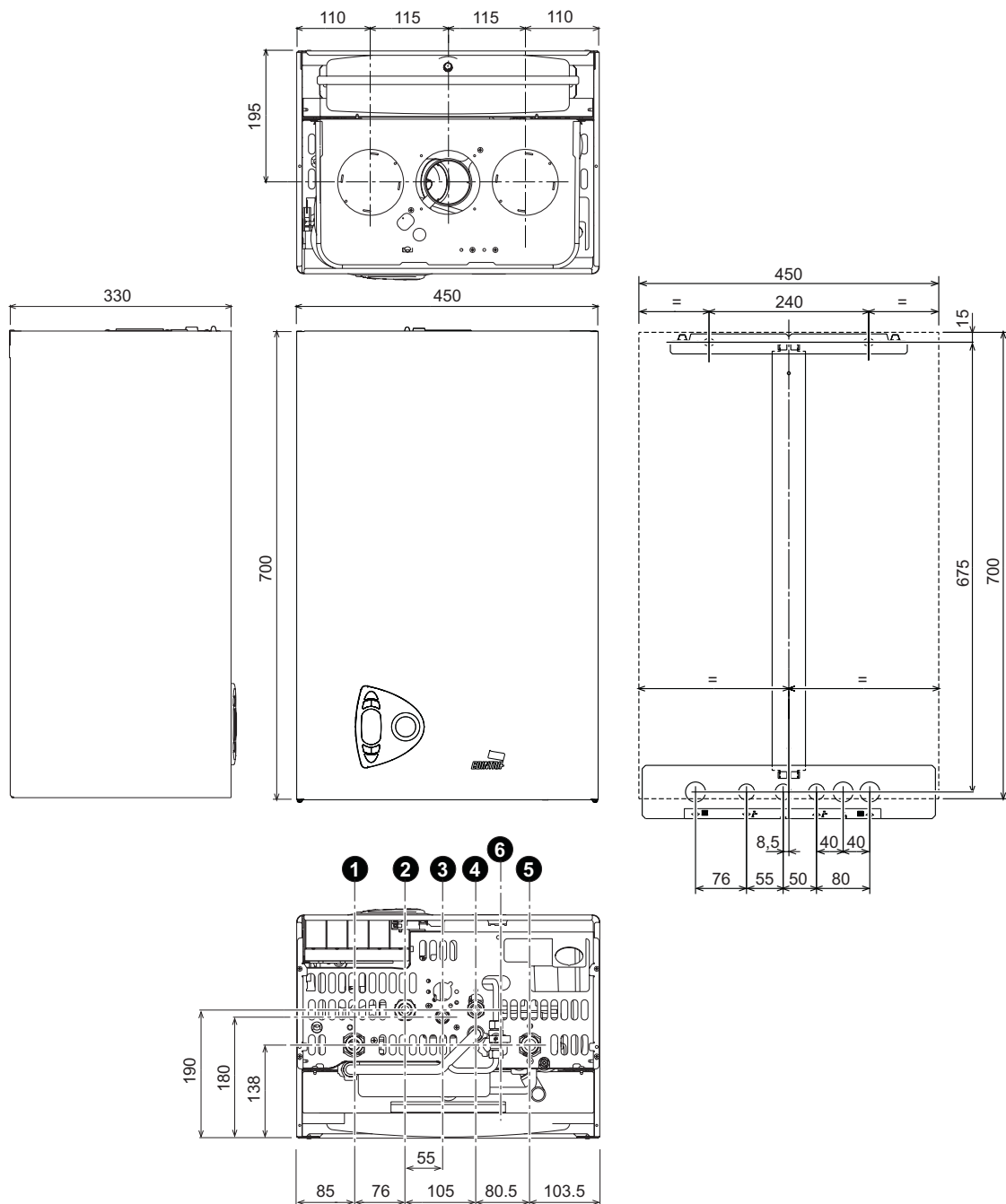
fig. 30 - Dimensiones y conexiones
