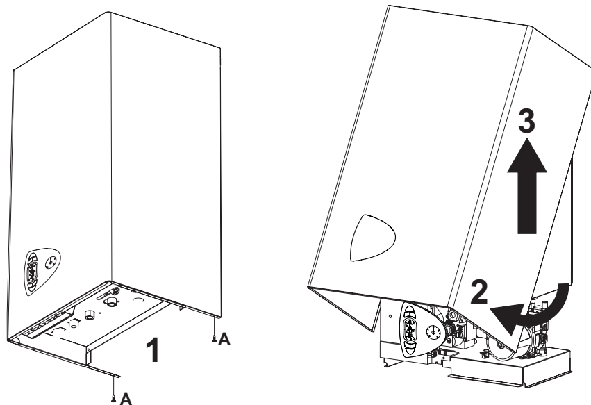
fig. 28 - Apertura de la carcasa
