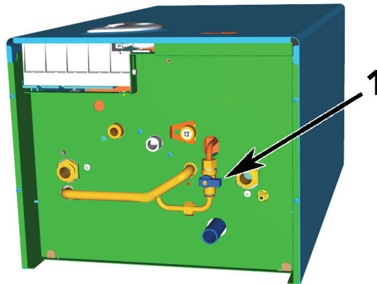
fig. 16 - Llave de carga
