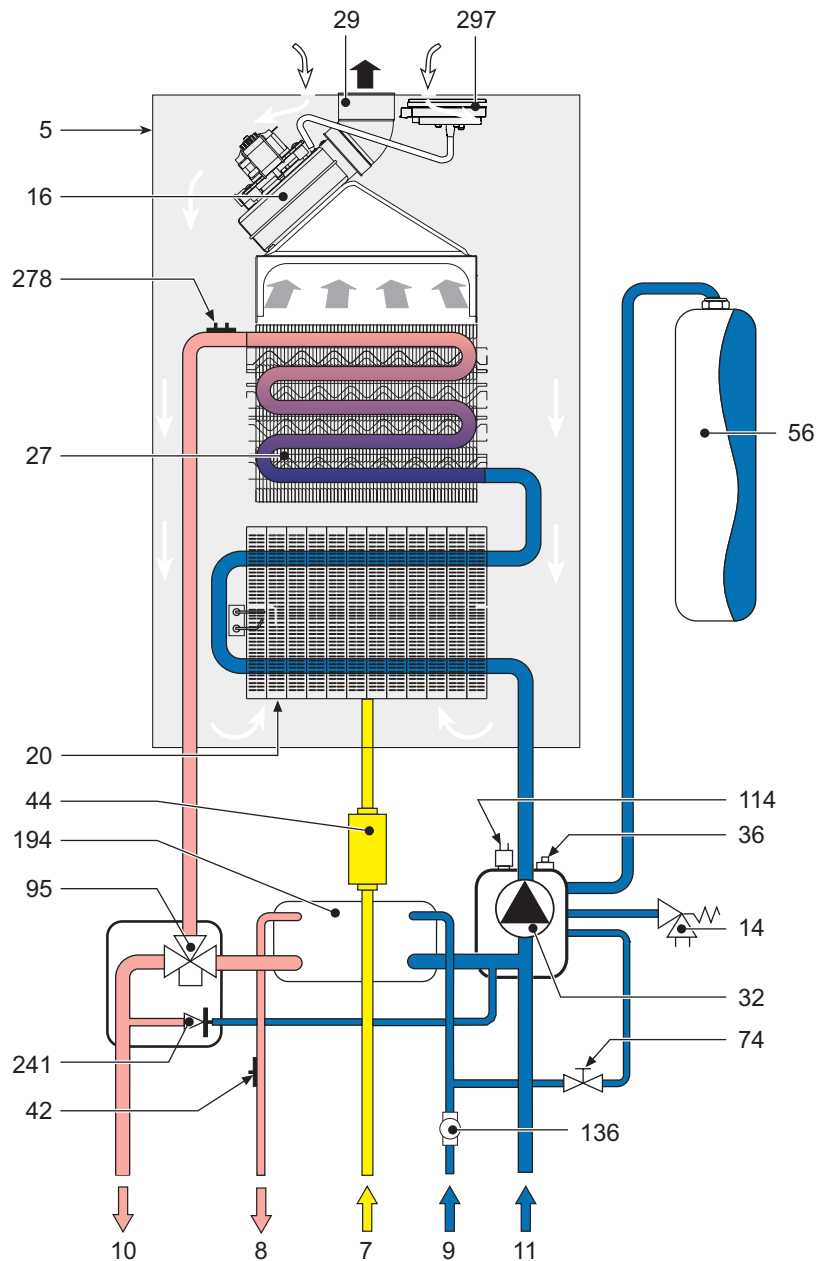
fig. 32 - Circuito hidráulico
